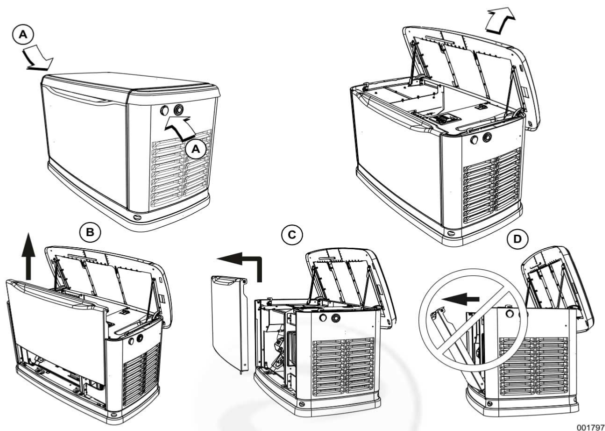
Рис. 3–1. Место бокового замка и снятие передней панели
