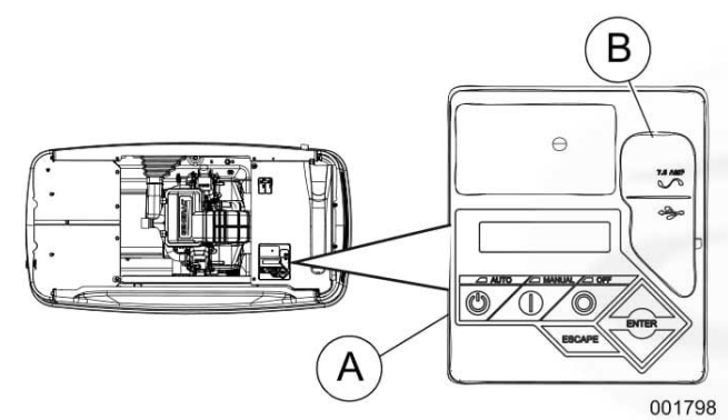
Рис. 3–5. Панель управления генератора
