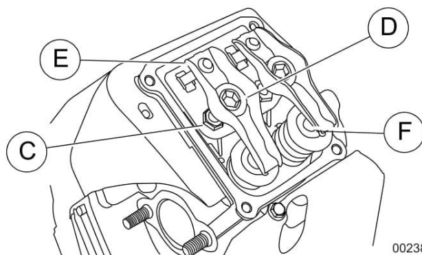
Рис. 4–5. Регулировка клапанного зазора
