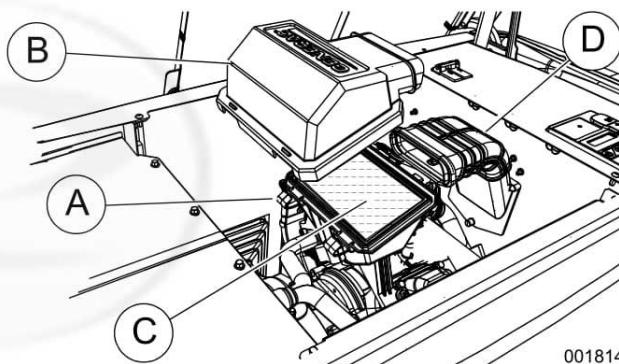
Рис. 4-3. Обслуживание воздухоочистителя
