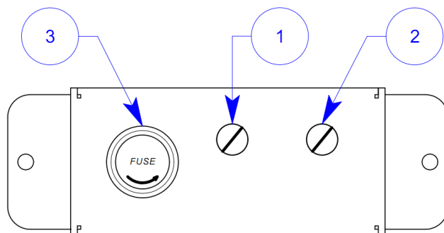
Рис. Блок настройки электрогенератора
